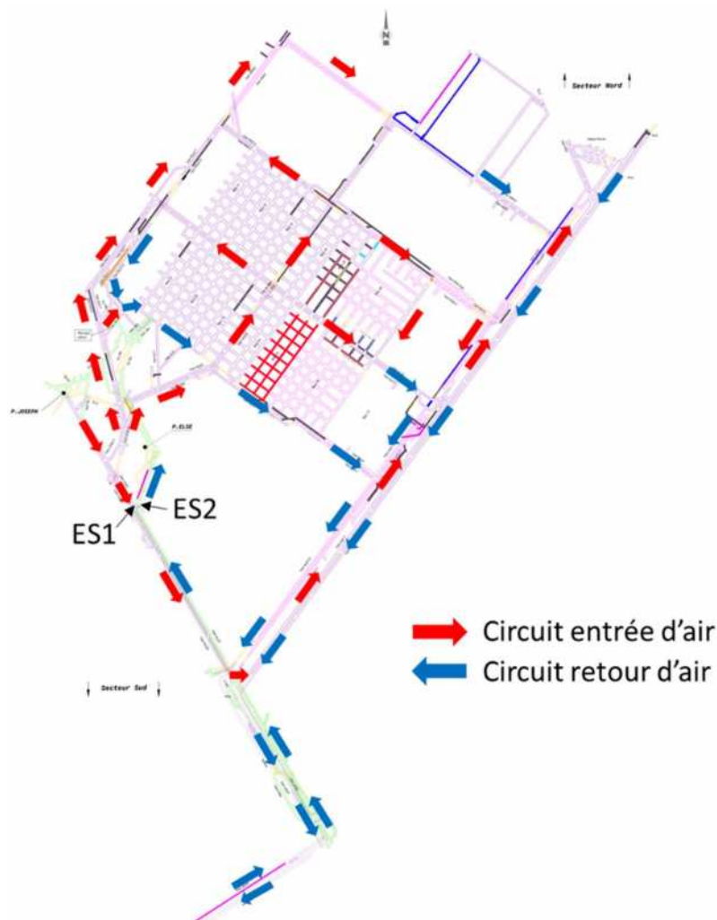
Figure 1 : Plan d'aéragé global de la mine
