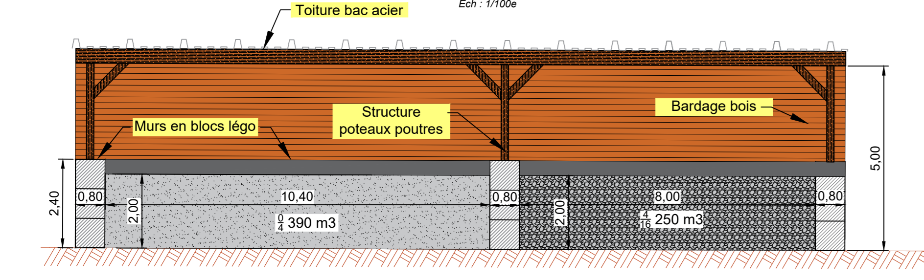
Coupe CC Ech : 1/100e
