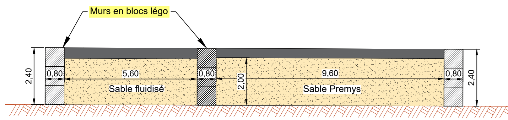
Coupe AA Ech : 1/100e
