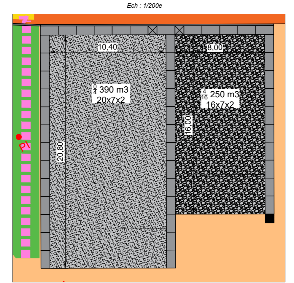
Vue en plan des casiers de granulats Ech : 1/200e
