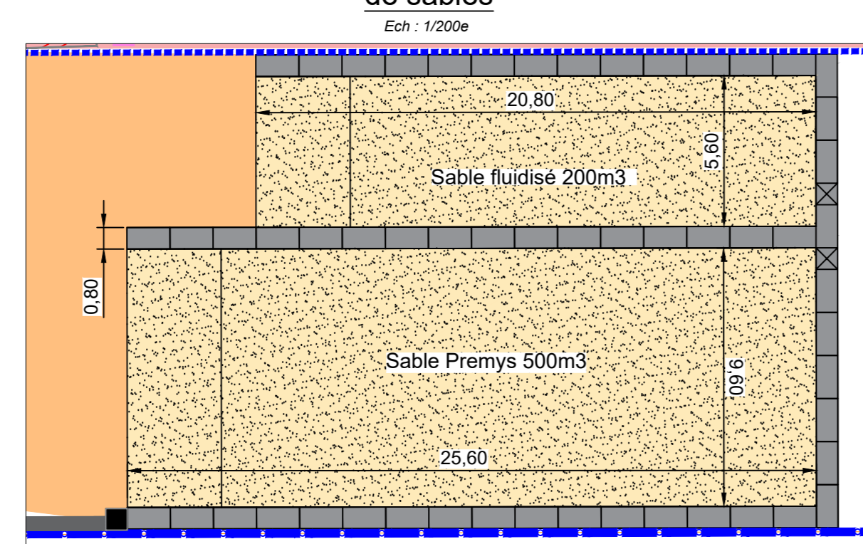
Vue en plan des casiers de granulats Ech : 1/200e
