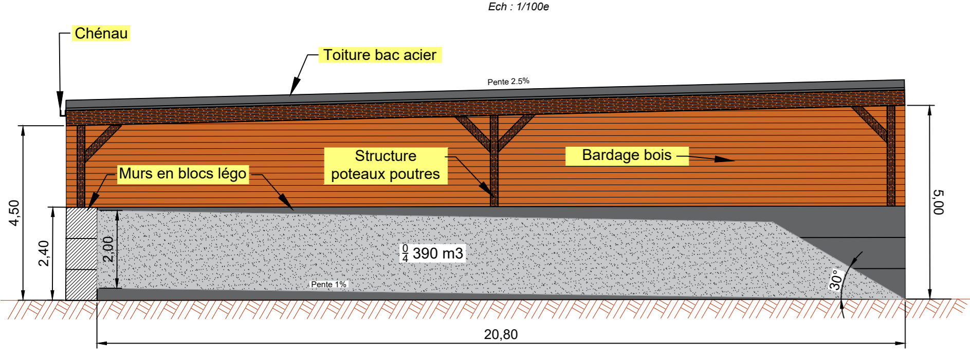
Coupe CC Ech : 1/100e
